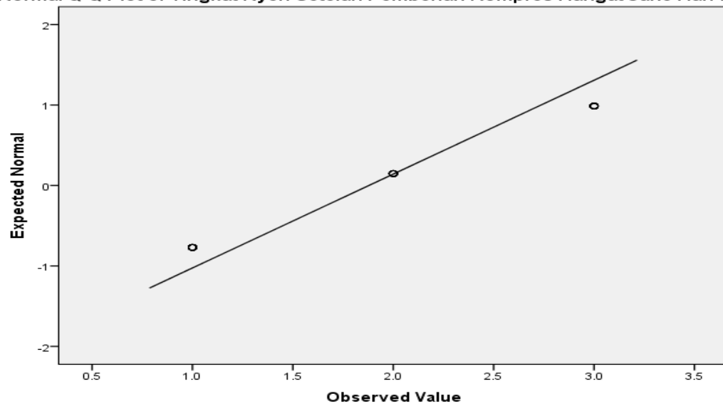
Normal Q-Q Plot of Tingkat Nyeri Setelah Pemberian Kompres Hangat Jahe Hari 7
