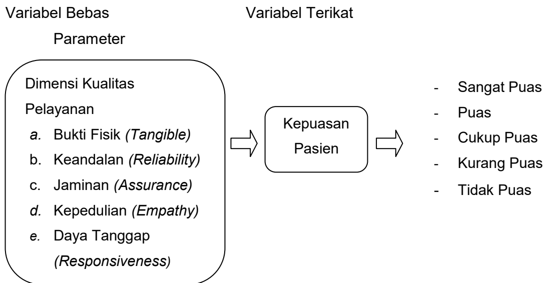
Gambar 2.1 Kerangka Konsep
