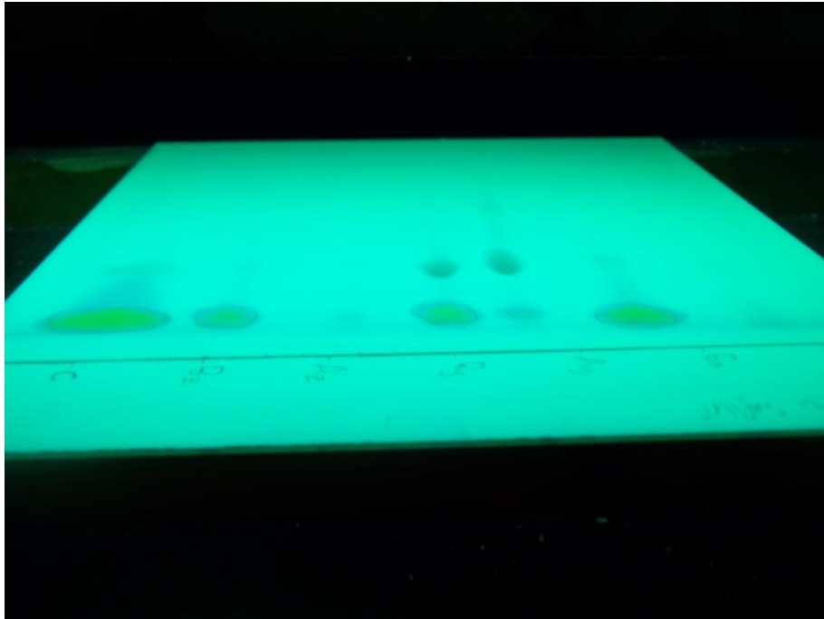
Gambar 8. Plat III dibawah sinar UV
