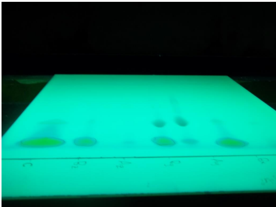
Gambar 7. Plat II dibawah sinar UV
