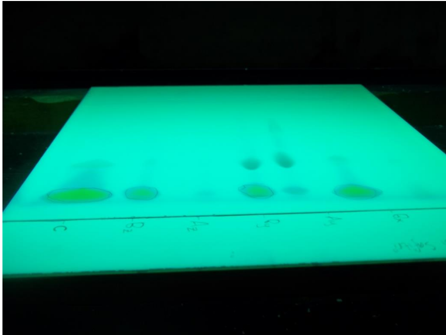
Gambar 6. Plat I dibawah sinar UV
